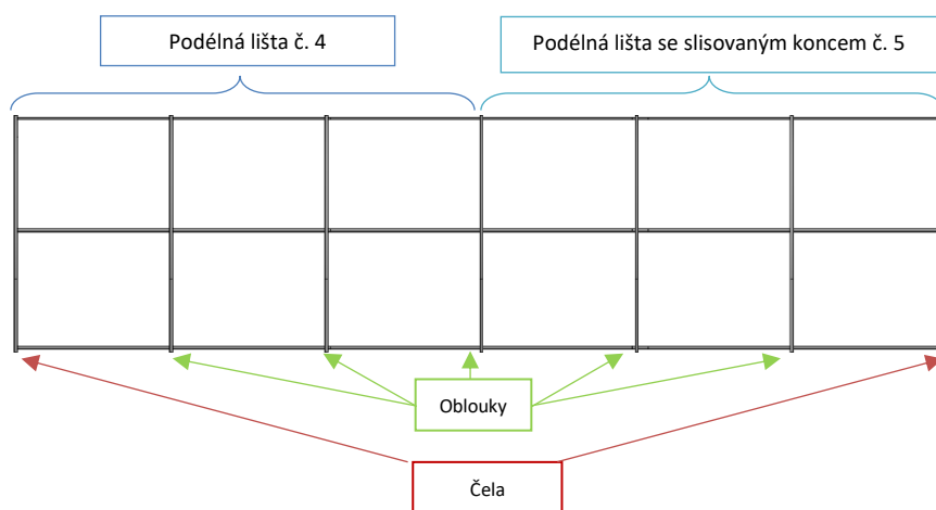
Příklad konstrukce 3,3 x 4 m
