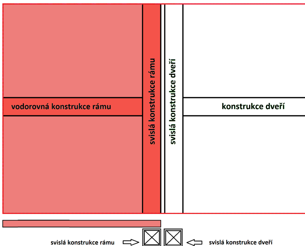
Obr. 5 – díl 1 posuňte až k úplnému okraji svislého rámu dveří
