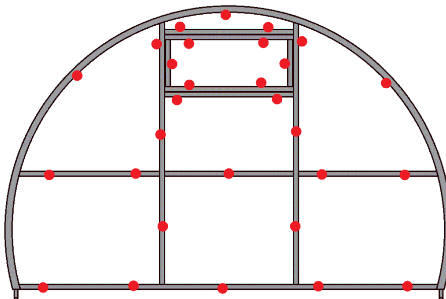
Obr. 7B – místa pro šroubu uchycující polykarbonát
