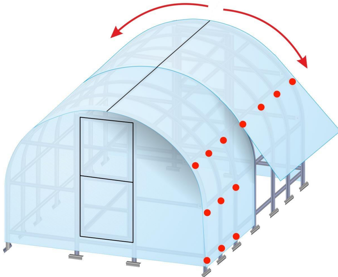
Ilustrativní obrázek umístění kotvicích šroubů pro polykarbonát
