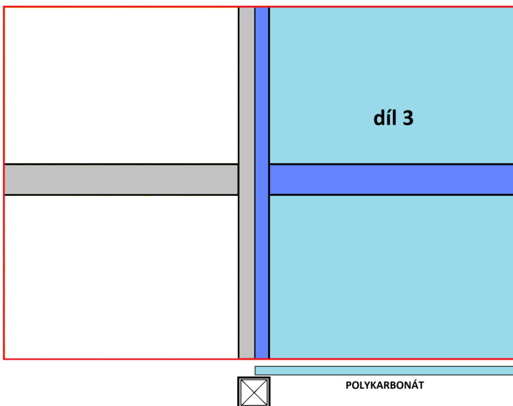
Obr. 3 – díl 3 posuňte doprostřed svislého nosného profilu
