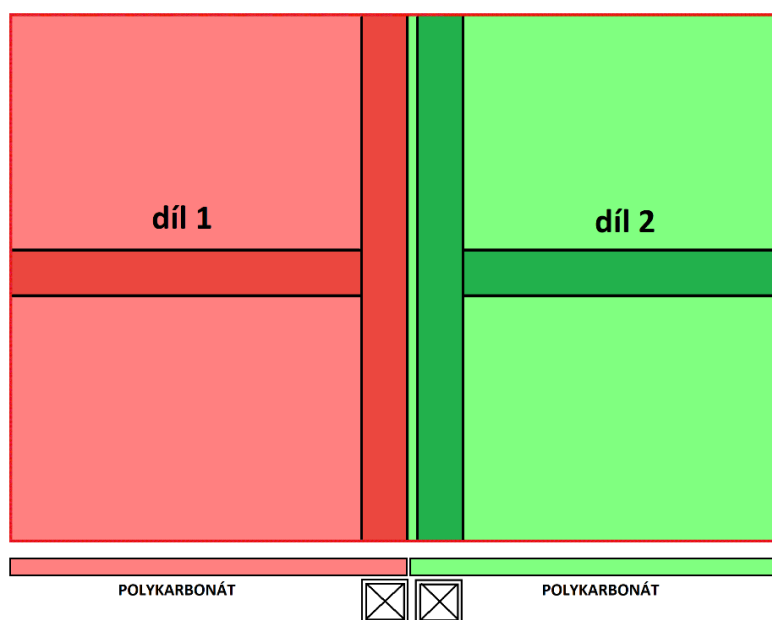
Obr. 6 – dva sousední díly 1 a 2
