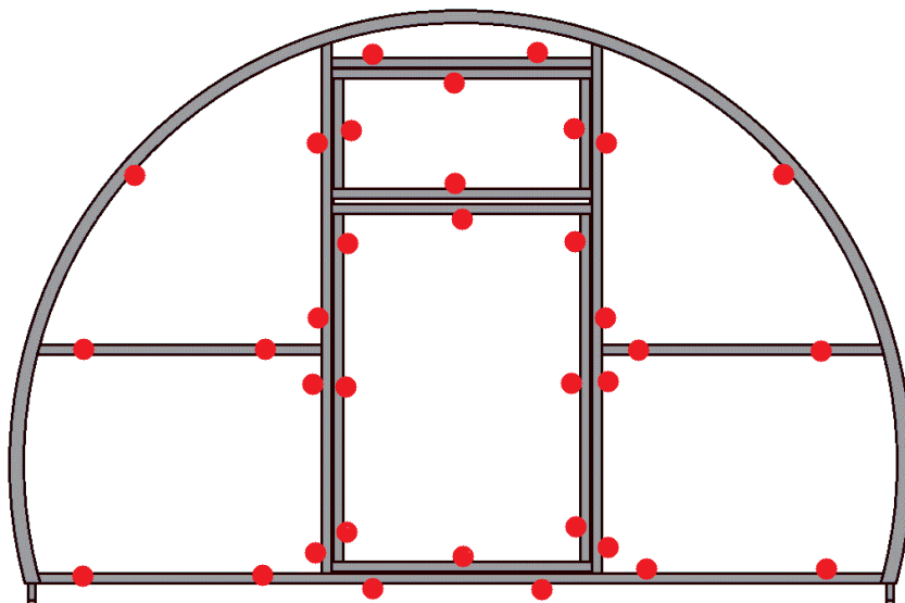
Obr. 6B – místa pro šroubu uchycující polykarbonát
